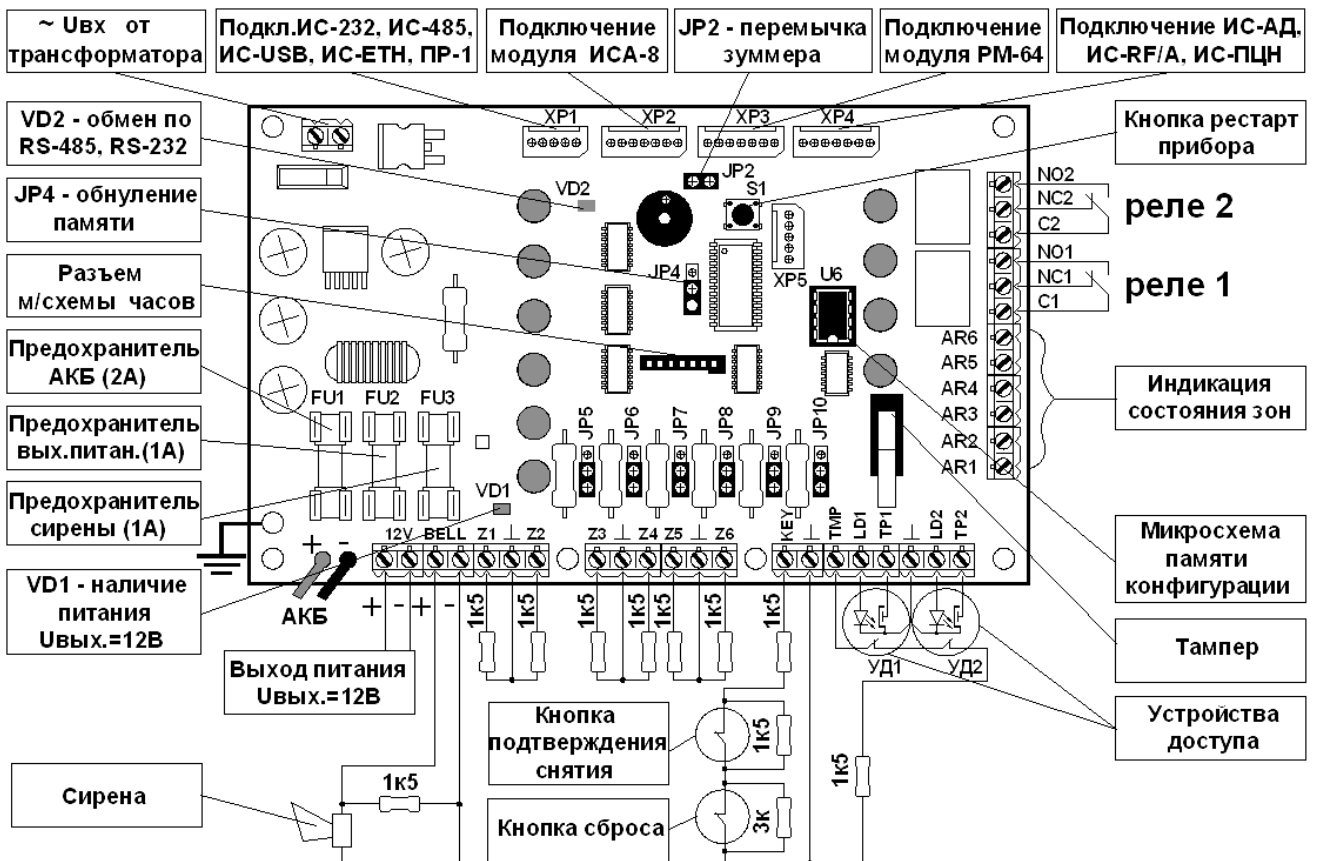
Рисунок 3 – Внешний вид платы управления прибора «А6» исполнения ППКОП А6-04
