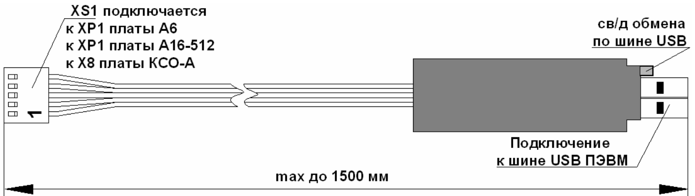
Рисунок 2 - Внешний вид модуля интерфейса ИС-USB
