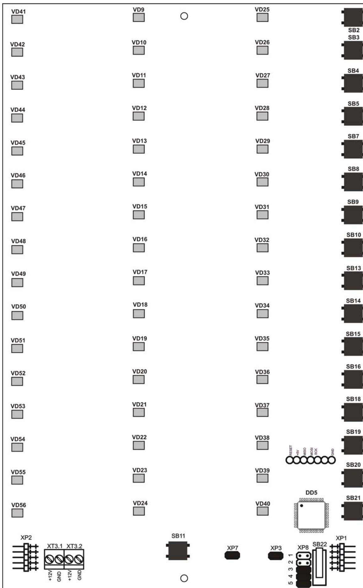
Рисунок 2.4.3 – Расположение разъемов и перемычек на плате модуля расширения
