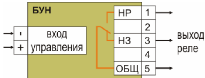
Рисунок 1. Подключение БУН
