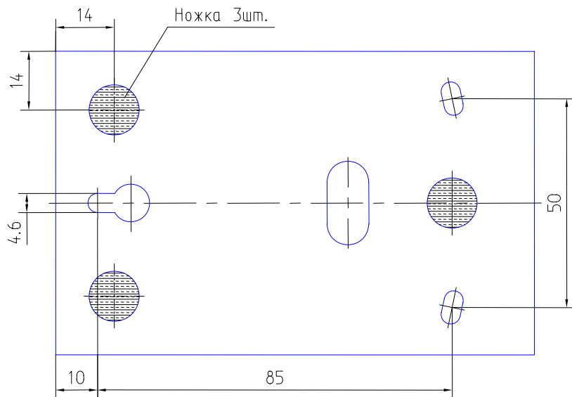
Схема установки приборных ножек при монтаже
