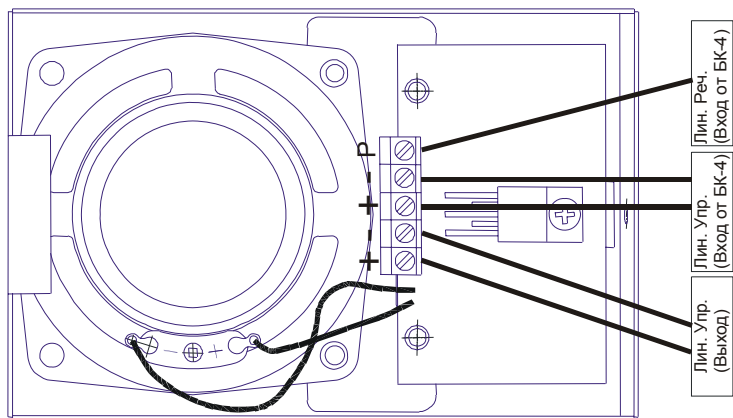
Схема подключения ОПК-1м
