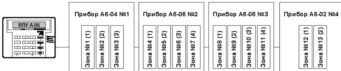
Рисунок 4 – Пример распределения зон в приборах и системе при объединении приборов «А6» при помощи ЖКИ клавиатуры ВПУ-А-06
